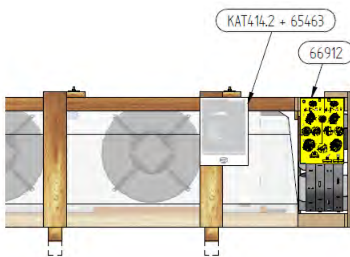
Деревянная упаковка для опции со стримером
